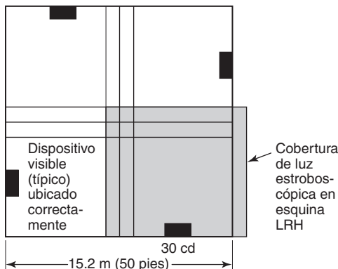
Figura A.18.5.5.4(c) Distribución del espaciamiento en salas — Correcto.
