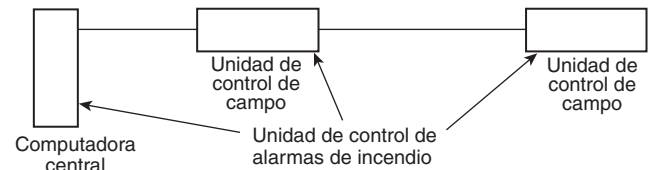
Figura F.3.5(a) Estilo 1.0 (Clase B).
