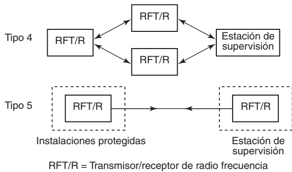
Figura F.3.14(c) Sistemas multiplex de radiofrecuencia de dos vías.
