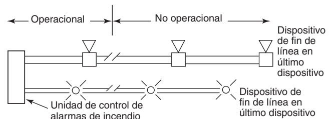
Figura F.2.12 Circuitos supervisados de aparatos de notificación audible y visible.
