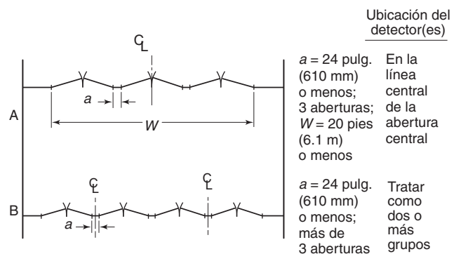
Figura 17.7.5.6.5.3(B) Requisitos de ubicación a \pm 24 pulg. (0.6 m) del/los detector/es para grupos de vanos de puertas.
